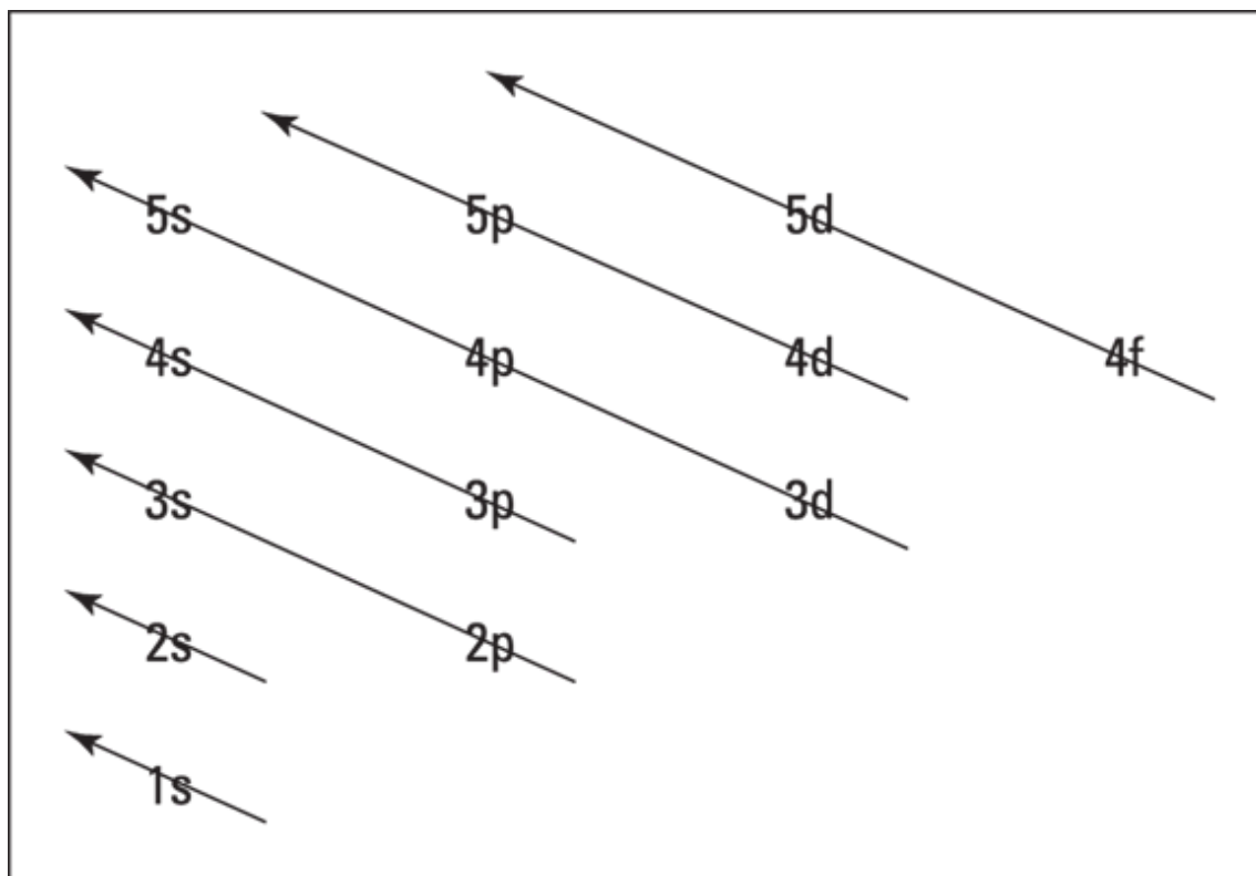
FIGURE 4-6: Aufbau filling chart.
